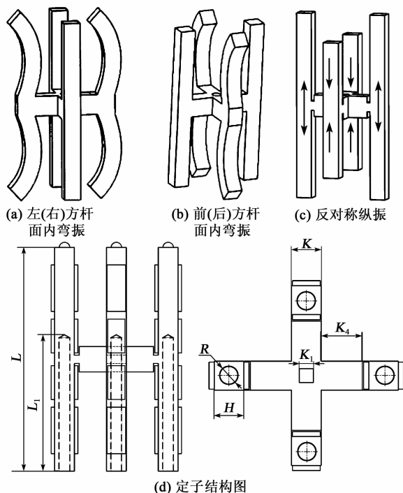
图 1 盆架形超声电机定子模型
