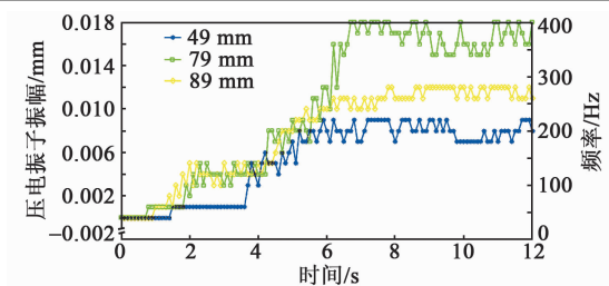
图7 压电驱动器振幅曲线图
