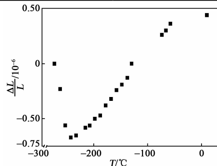
图 1 石英材料 \Delta L/L 与 T 的关系图
