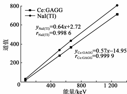
图6 线性度对比
