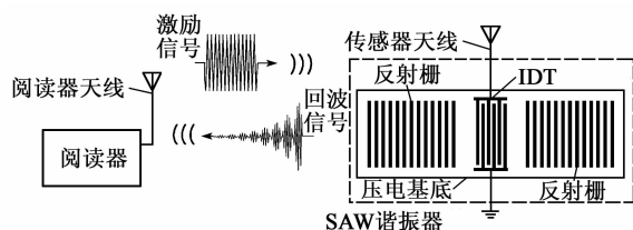
图 1 SAW 扭矩检测系统
