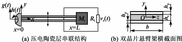
图 1 悬臂式压电振动能量采集器结构简图
