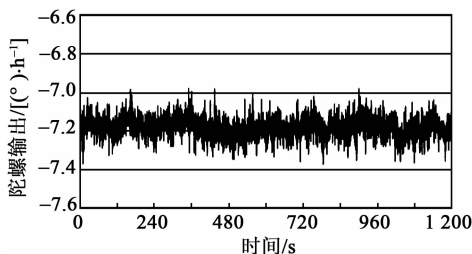
图3 低噪声半球陀螺的噪声
