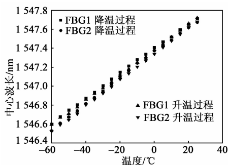
图5 FBG1、2 升、降温过程中中心波长的位置图
