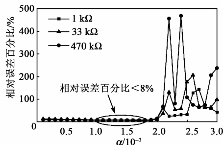
图5 模型与实验结果相对误差百分比
