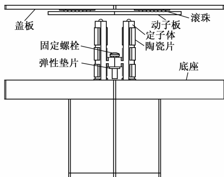
图 10 盆架形定子电机装配结构
