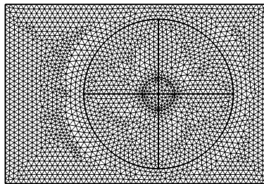
图 2 声学黑洞板结构网格划分图
