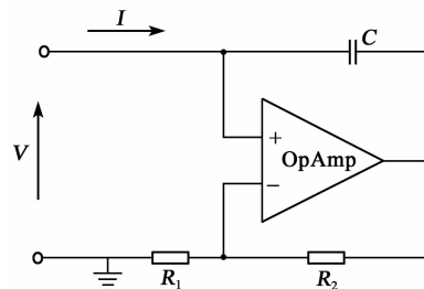
图2 负电容合成电路
