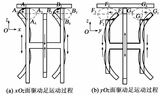
图3 定子驱动足运动轨迹
