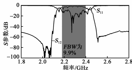
图8 LiNbO 3 -on-SiC SAW 滤波器的测试结果
