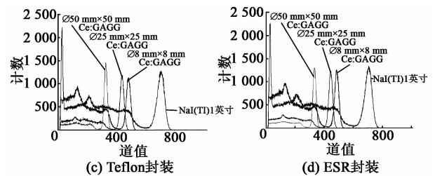
图 4 不同反射层封装材料能谱图
