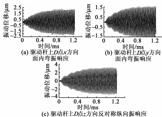
图7 驱动足沿x、y、z方向的振动响应
