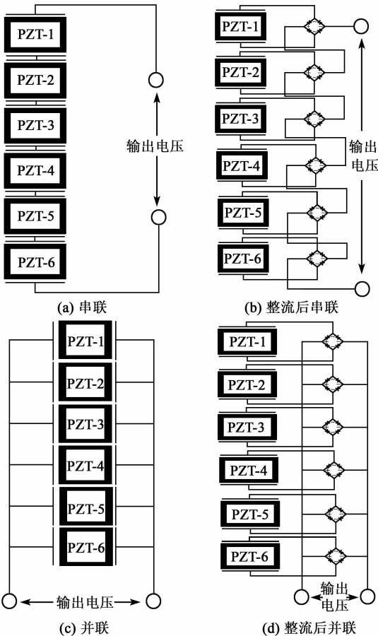
图 6 不同电路连接组合图
