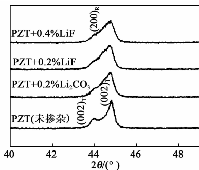
图2 图1的XRD放大图
