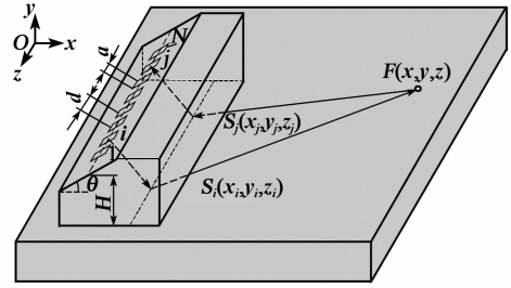
图1 相控阵表面波延时计算原理图
