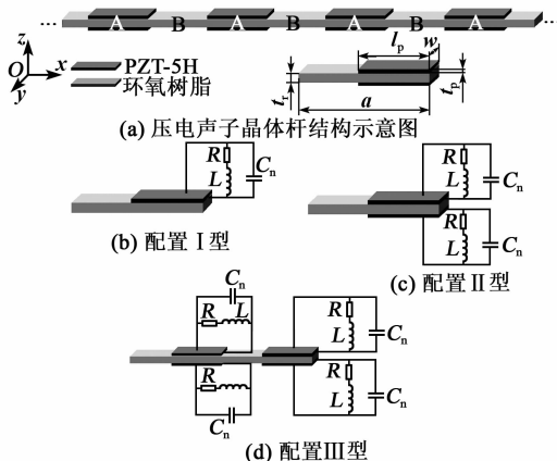
图1 压电声子晶体杆及3种元胞配置示意图
