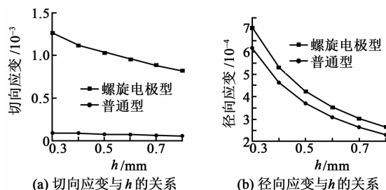
图 13 应变与 h 的关系
