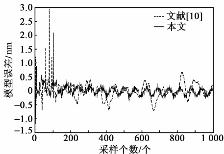
图 9 本文与文献[10]建模误差对比
