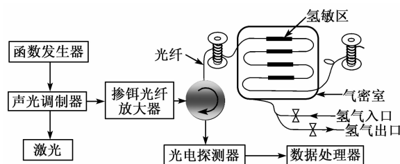
图 6 \Phi -OTDR 检测系统原理图
