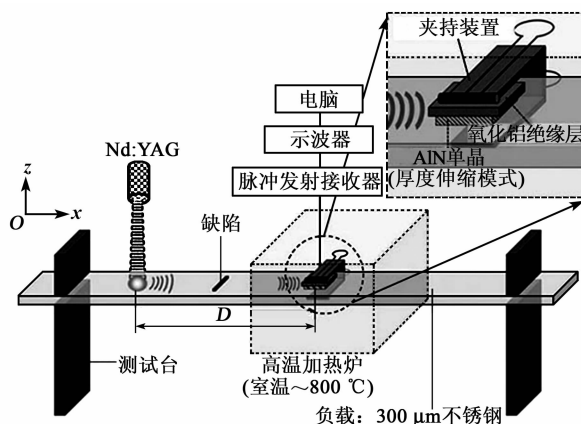
图9 AlN基压电换能器接收性能测试装置
