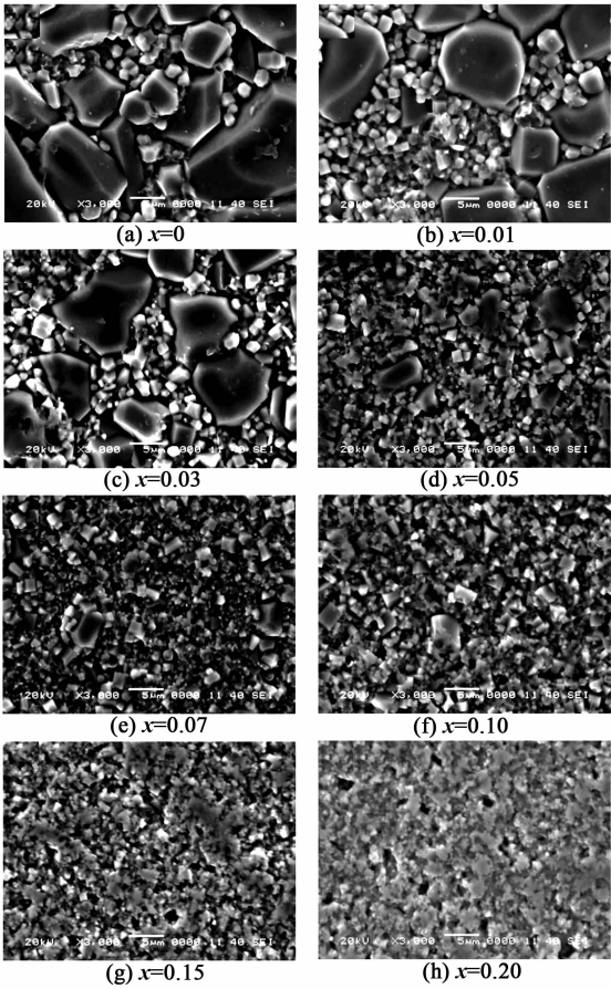
图 2 (\text{Ca}_{0.97}\text{Ba}_{0.03})\text{Cu}_3\text{Ti}_{4-x}\text{Nb}_x\text{O}_{12} 陶瓷的表面微观形貌图
