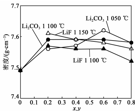
图4 烧结温度及 x 、 y 不同时样品的密度图
