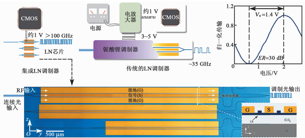
图2 集成 LNOI 电光调制器
