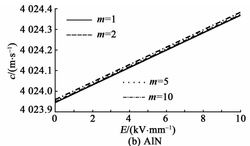
图 2 ZnO、AlN 材料中 c 与 E 的关系
