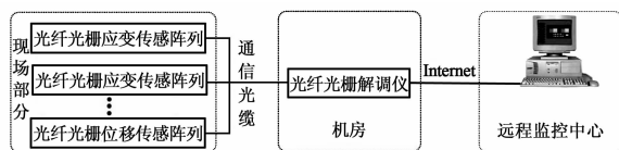
图 1 基于准分布式光纤光栅传感网络的电梯钢架结构监测系统结构示意图
