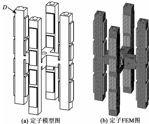
图 4 定子构型图
