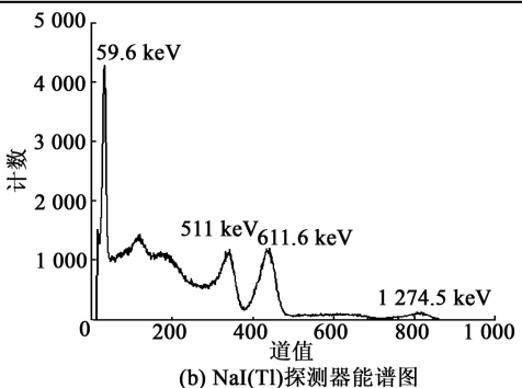
图 5 探测器线性度测试能谱图
