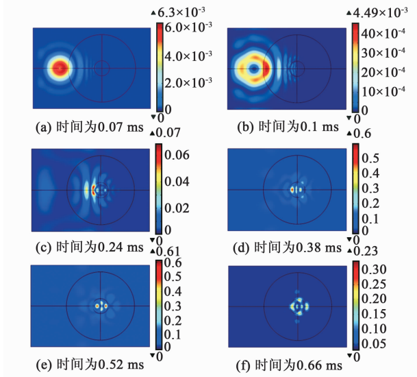
图 4 时域下动能密度
