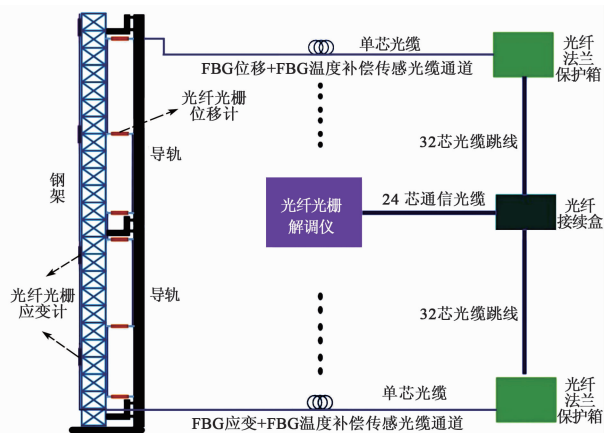
图 3 准分布式光纤光栅传感网络设计与安装
