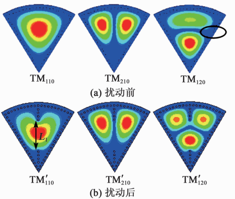
图 2 谐振器电场分布
