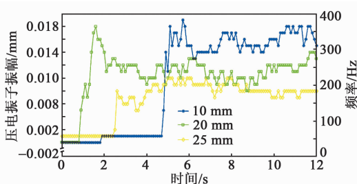
图9 压电振子位移曲线图
