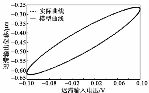
图3 f = 50 Hz时实际与模型输出曲线
