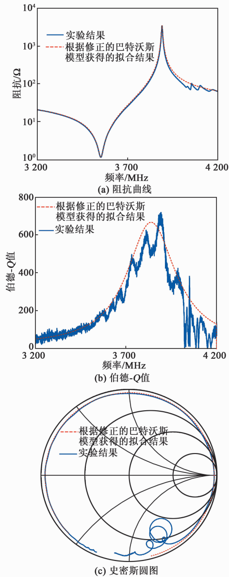
图6 3.5 GHz LLSAW谐振器的检测拟合特性
