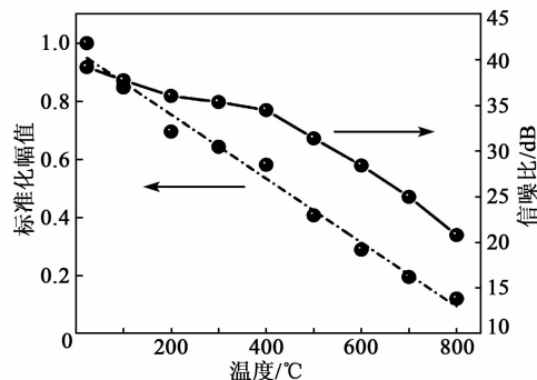
图10 S_0 波的标准化振幅和对应 S_0 波的信噪比
