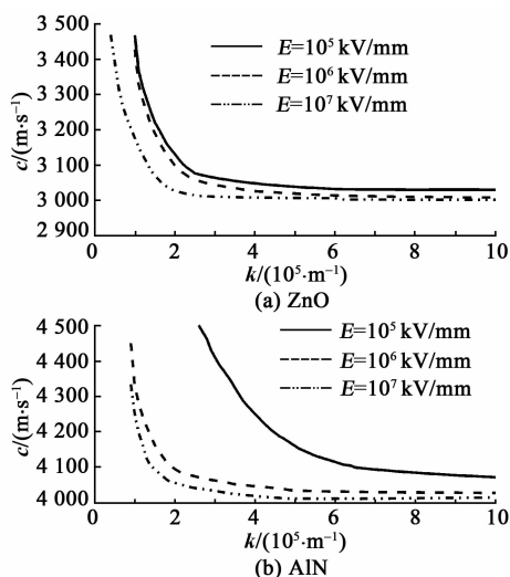
图 3 静电场作用下 ZnO、AlN 材料的频散曲线
