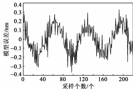
图 6 f=50 Hz 时实际模型误差曲线
