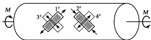
图 2 传感器粘贴方案示意图
