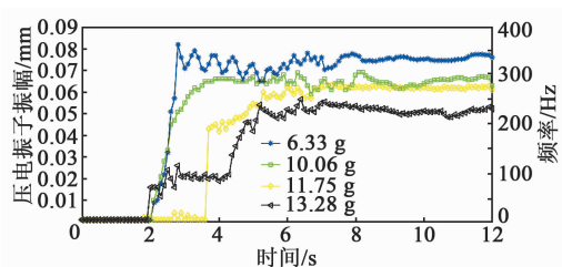
图5 压电驱动器振幅曲线图
