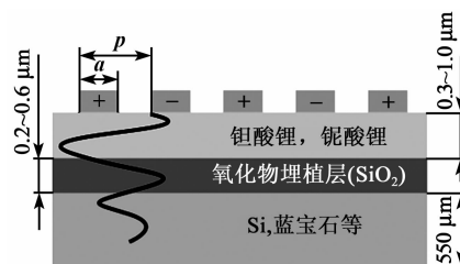
图4 采用 Smart-Cut 技术制备的 SAW 器件用标准波导/材料叠层
