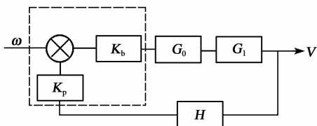
图1 控制系统框图
