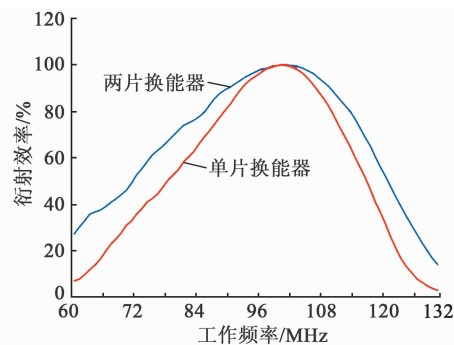
图8 衍射效率归一化
