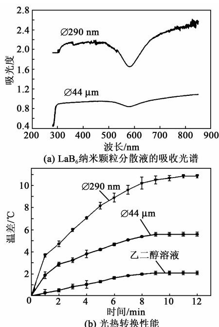
图2 w(\text{LaB}_6) = 0.15\% 时, \text{LaB}_6 纳米颗粒分散液的吸收光谱及光热转换性能
