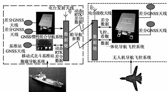
图 1 基于 SINS/北斗 RTK 导航系统组成框图
