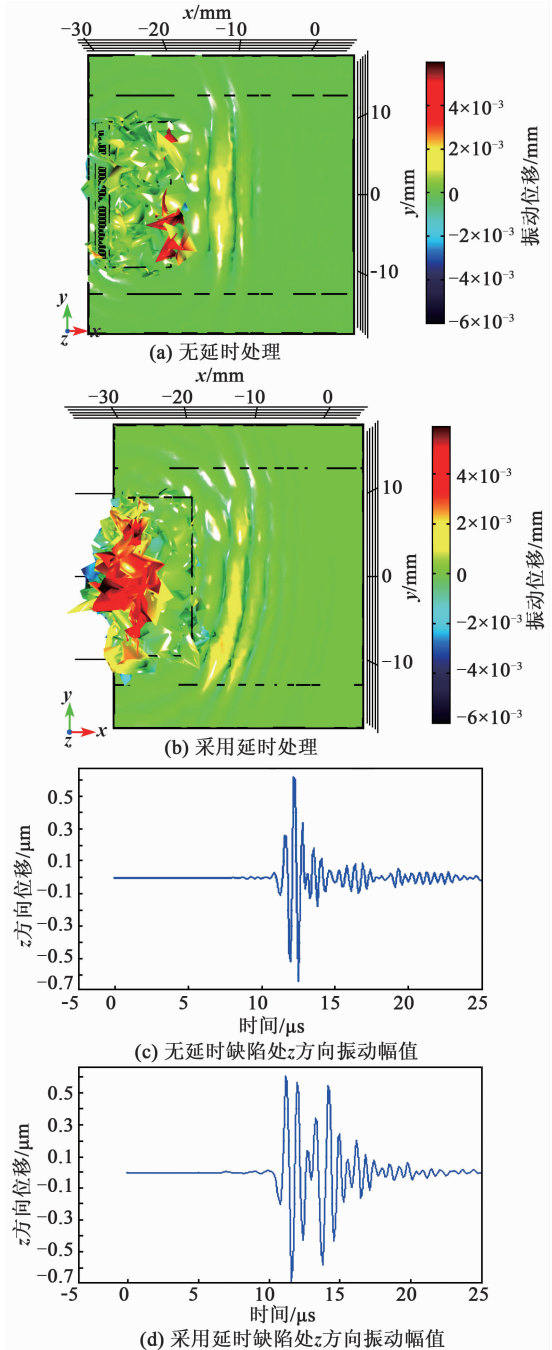
图5 相控阵激励仿真结果
