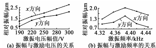
图9 盆架形定子驱动足振动调节特性
