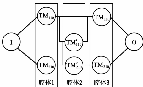
图 5 电路拓扑结构
