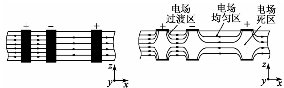
图7 电场分布图
