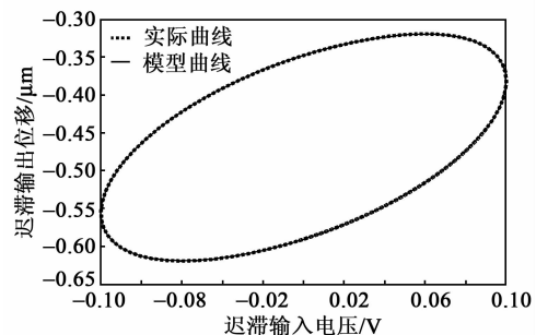
图4 f = 100 Hz时实际与模型输出曲线
