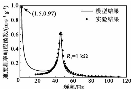
图3 模型结果与实验结果对比
