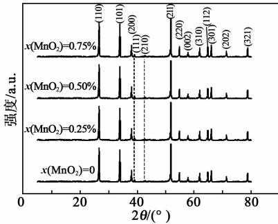
图 2 \text{SnO}_2\text{-ZnO-MnO}_2\text{-Ta}_2\text{O}_5 压敏陶瓷的 XRD 图谱
