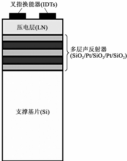
图5 日本村田公司提出的LLSAW波导结构 [5]
