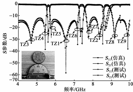
图10 滤波器仿真和测试结果
