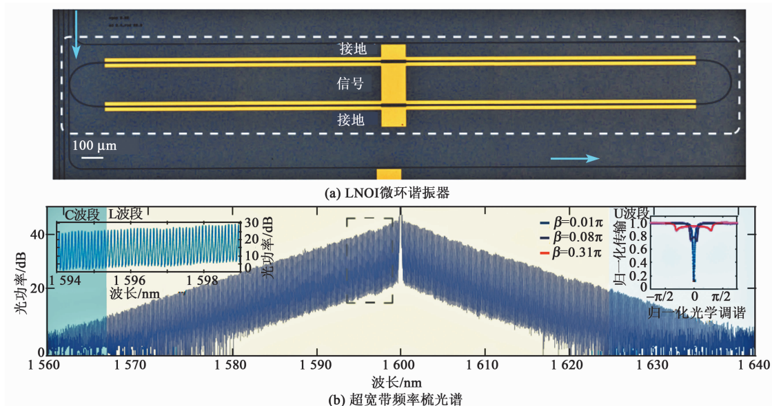
图6 集成电光频率梳
