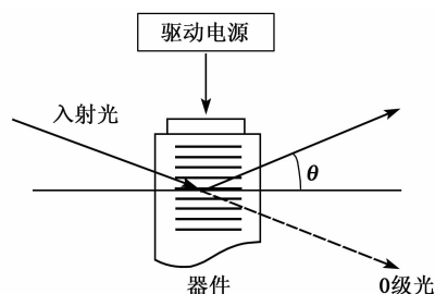
图5 声光器件衍射原理图
