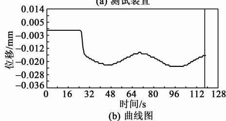
图 2 驱动器振幅测试装置及曲线图
