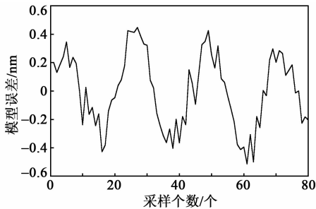
图 7 f=100 Hz 时实际模型误差曲线
