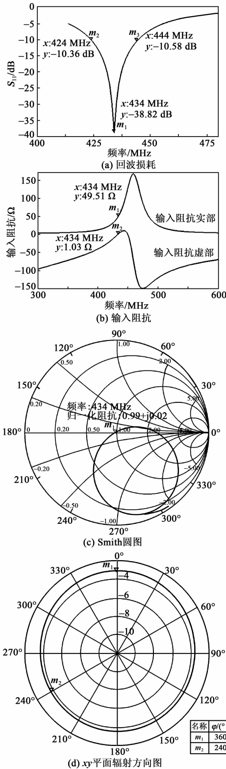
图8 根据优化的天线结构参数得到的仿真结果
