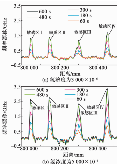
图7 准分布式光纤氢传感器对氢气响应特性
