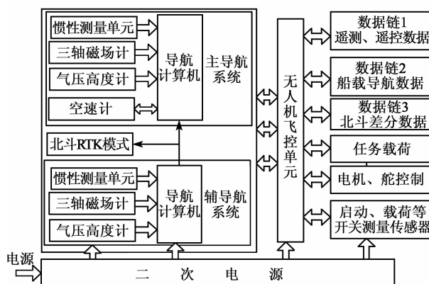
图 2 无人机一体化导航飞控系统组成框图
