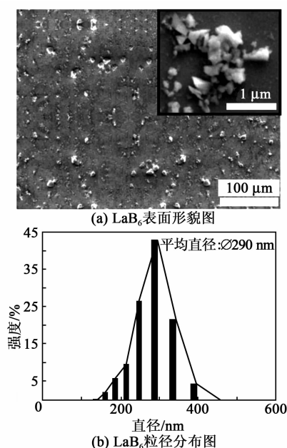
图1 \text{LaB}_6 表面形貌及粒径分布图
