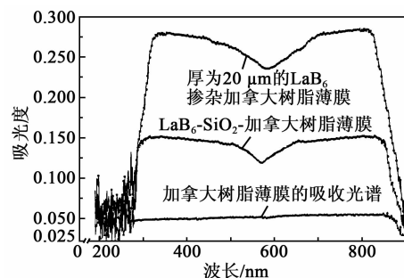
图3 涂覆膜吸收光谱
