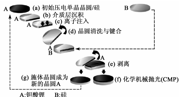
图2 Smart-Cut技术的原理及POI基片的制作工艺流程
