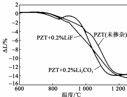
图3 掺杂 LiF 、 Li_2CO_3 样品的烧结收缩曲线图
