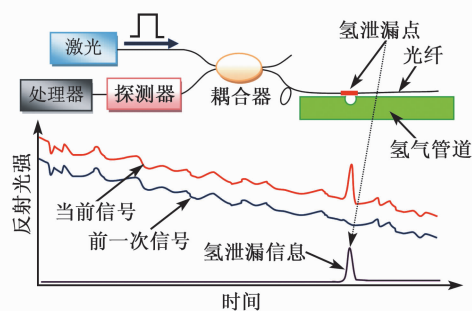
图1 \Phi -OTDR 氢气泄漏检测原理示意图
