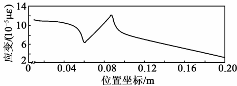
图 4 脱粘路径应变分布
