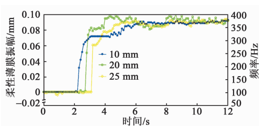
图10 柔性薄膜位移曲线图
