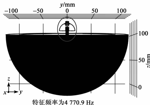
图 3 PML 仿真模型总体示意图
