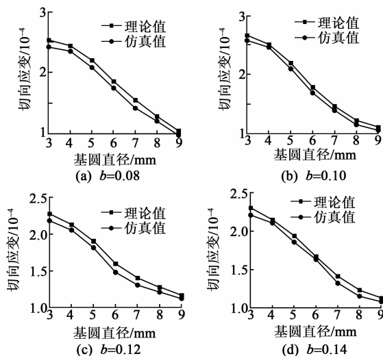
图 10 切向应变与基圆直径的关系
