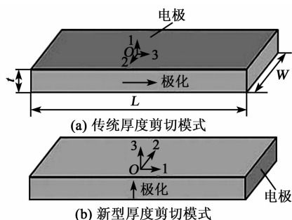
图1 传统与新型厚度剪切模式
