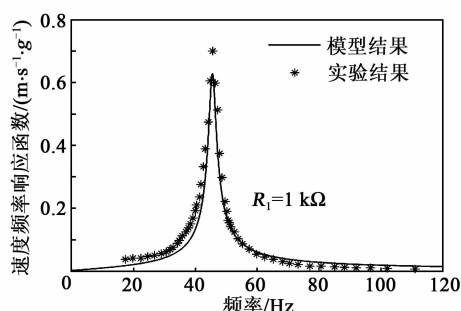
(a) 引入单项 \alpha 的速度频率响应
