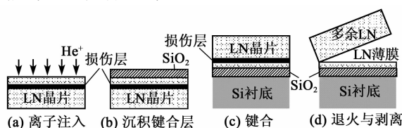
图1 LNOI制备流程
