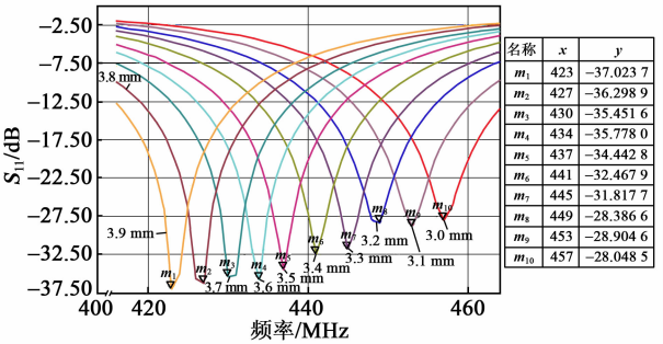
图 7 辐射体宽度参数化扫描回波损耗变化
