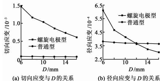
图 12 应变与压电圆盘直径的关系
