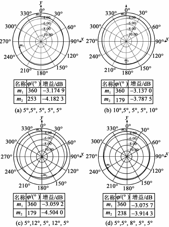
图 5 辐射体段不同重叠角度对应的 xy 平面辐射方向图
