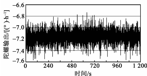
图2 常规半球陀螺的噪声
