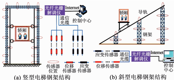
图 2 准分布式光纤光栅传感网络在竖型和斜型电梯钢架结构中的设置
