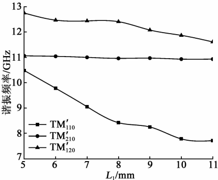
图 3 不同 L_1 参数对谐振器频率的影响
