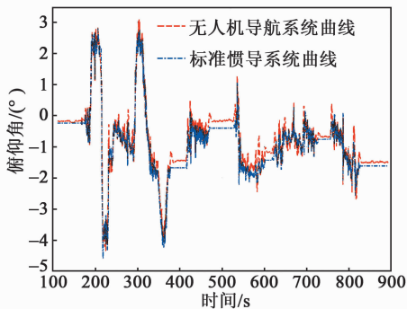
图 7 导航系统与标准惯导俯仰对比曲线
