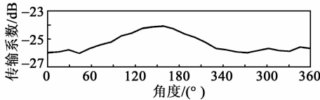
图 11 天线全向性测试结果
