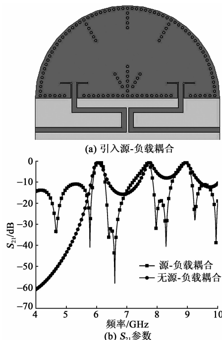
图 8 引入源-负载耦合前后的 S_{21} 对比
