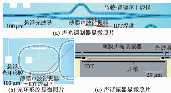
图 5 悬浮 LN 薄膜上的集成 AO 器件
