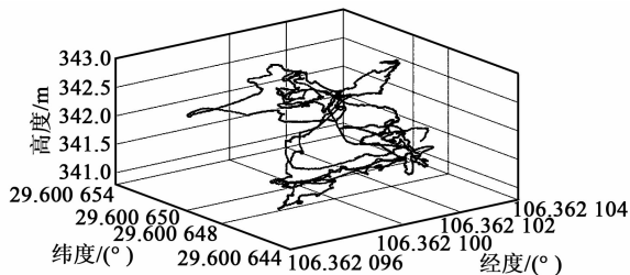
图 3 动 RTK 地理系下导航系统定位曲线
