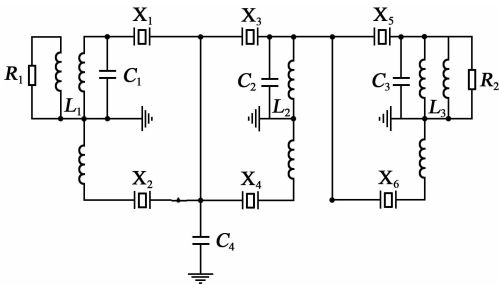
图 3 晶体滤波器电路图
