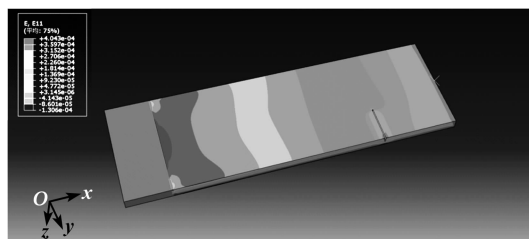
图 2 长度方向应变场
