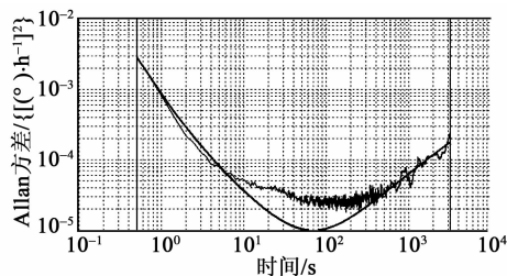
图5 低噪声半球陀螺的Allan方差曲线
