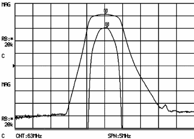
图 4 晶体滤波器通带响应曲线
