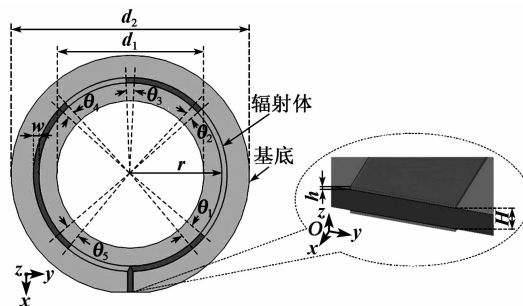
图 3 分段环状天线结构
