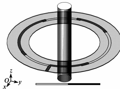
图 4 分段环状天线和转轴模型
