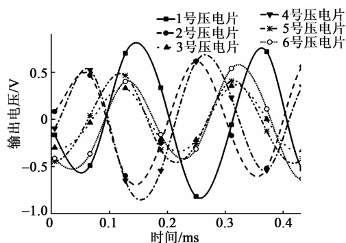
图9 单个压电片输出电压幅值
