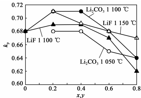
图7 烧结温度及 x 、 y 不同时样品的 k_p 图
