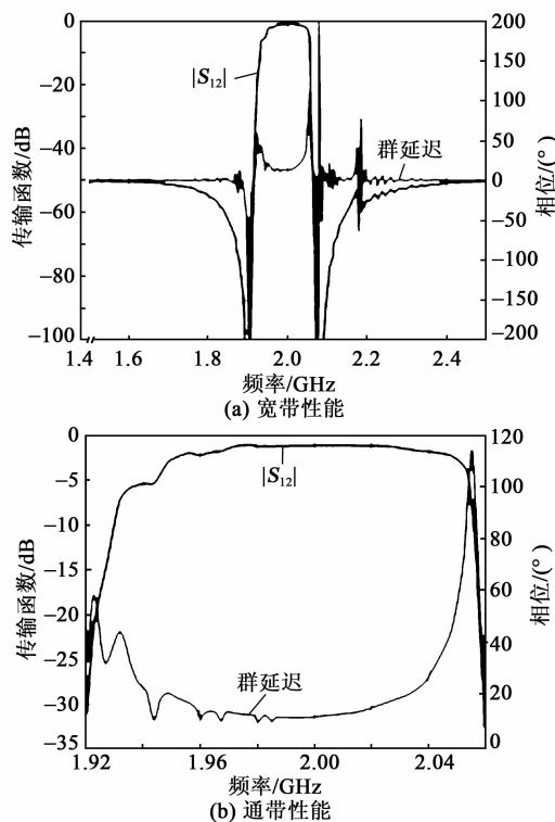
图 10 POI 基片 2 GHz SAW 滤波器的传输函数及群延迟
