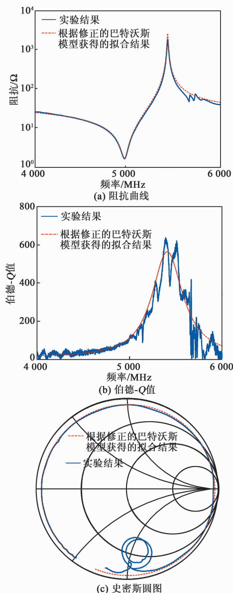
图7 5 GHz LLSAW 谐振器的检测拟合特性
