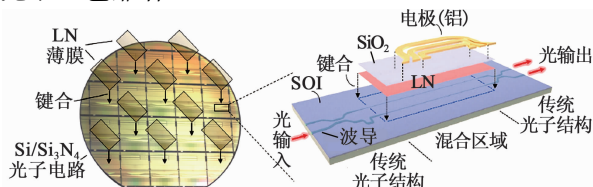
图 3 3 dB 电调制带宽大于 100 GHz 的 Si/LN 混合集成电光调制器
