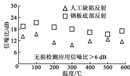
图8 室温至 600\text{ }^{\circ}\text{C} 时, \text{GaPO}_4 基压电换能器信噪比数值变化示意图
