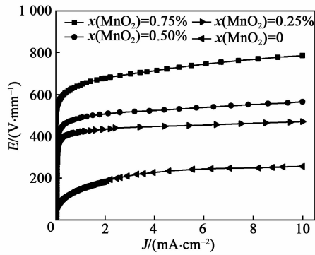
图 3 \text{SnO}_2\text{-ZnO-MnO}_2\text{-Ta}_2\text{O}_5 压敏陶瓷的 E\text{-}J 特性曲线
