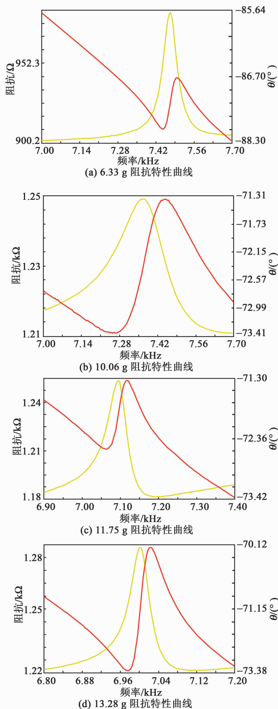
图3 不同配重质量驱动器阻抗图
