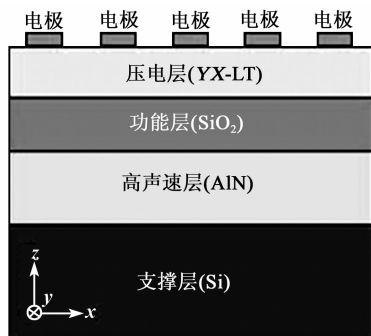
图3 村田公司 I. H. P. SAW 的基本结构
