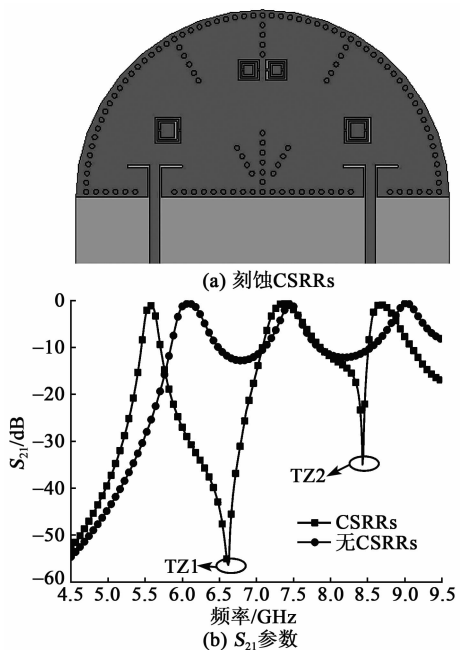
图 7 刻蚀两对 CSRRs 前后的 S_{21} 对比
