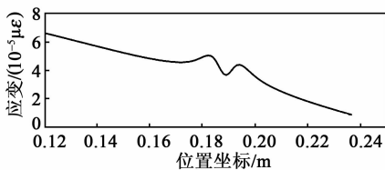
图 5 裂纹路径应变分布
