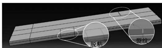
图 1 有限元模型
