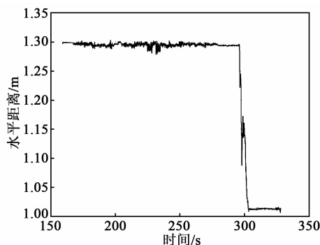
图 9 动态 RTK 相对定位水平距离曲线
