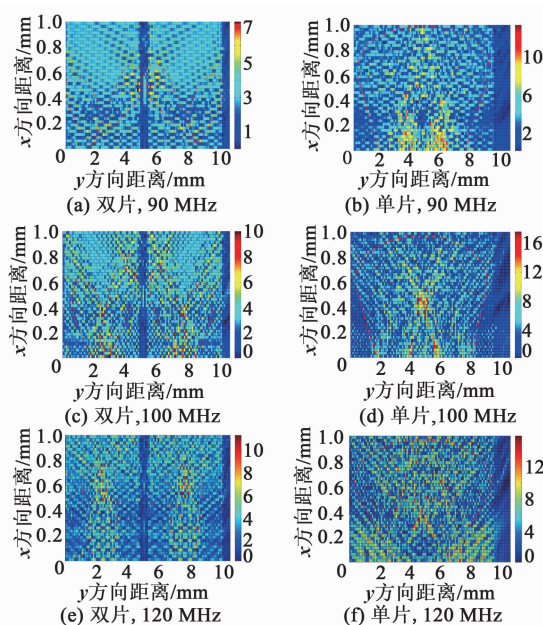
图7 中心频率 100 MHz 辐射声场分布仿真图
