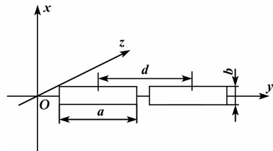
图 4 换能器安装示意图
