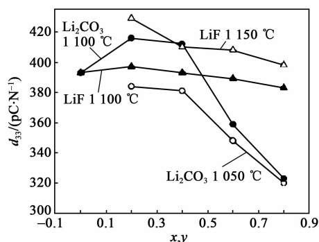
图6 烧结温度及 x 、 y 不同时样品的 d_{33}
