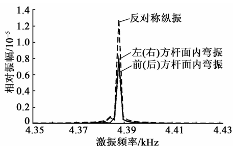
图6 定子振动频率特性曲线
