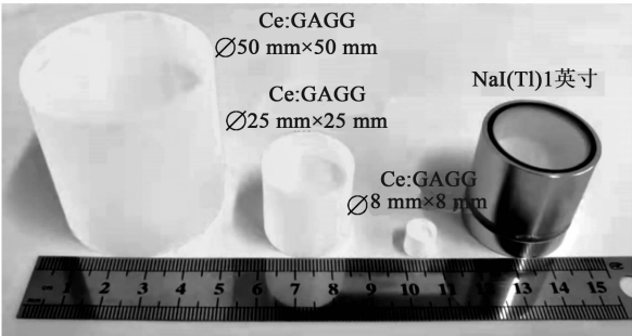
图 2 闪烁体图片
