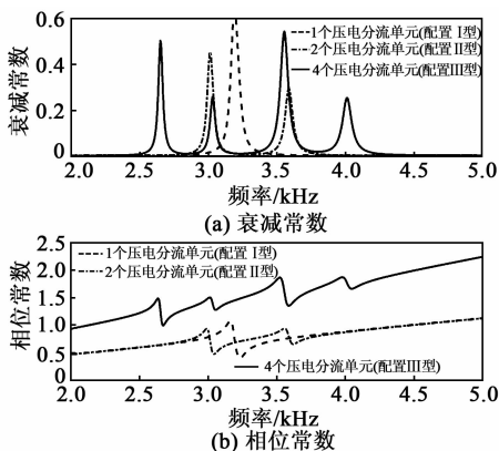
图4 3种元胞配置下压电声子晶体杆的带隙结构
