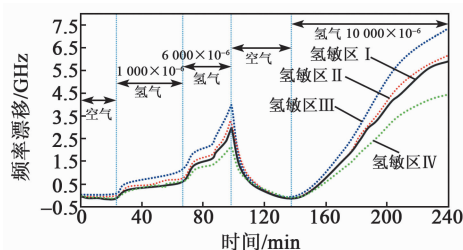
图8 光纤氢传感器在 240 min 内对氢气的连续响应特性
