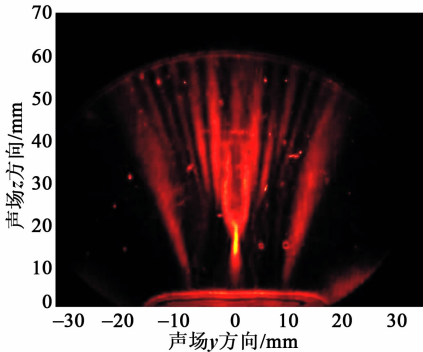
图 8 声场聚焦于(0, 0, 15 mm)的 Schlieren 像
