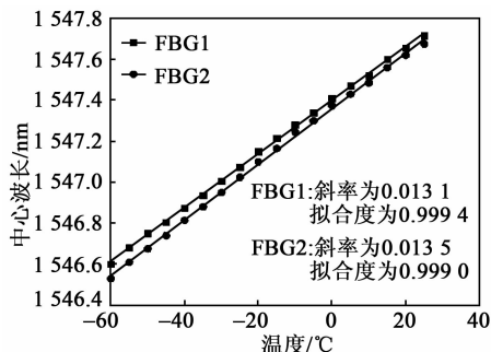
图6 FBG1、2 的波长漂移线性拟合图
