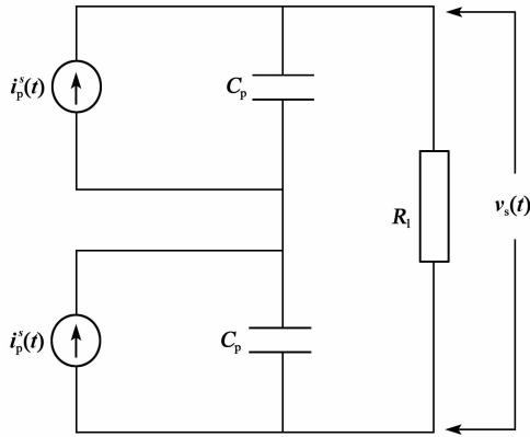
图2 电路简图
