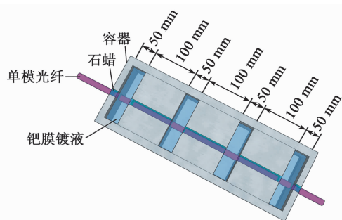
图2 氢敏分布式光纤传感器制备容器结构示意图
