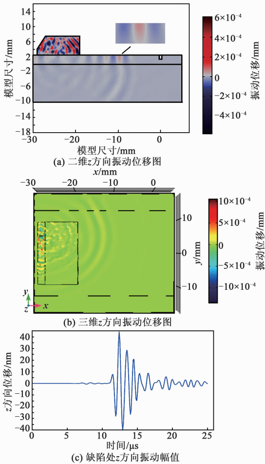
图3 单探头激励仿真结果
