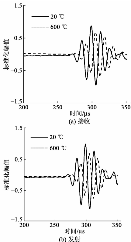
图 5 LN 基压电换能器在室温 and 600 °C 下接收和发射信号的幅值
