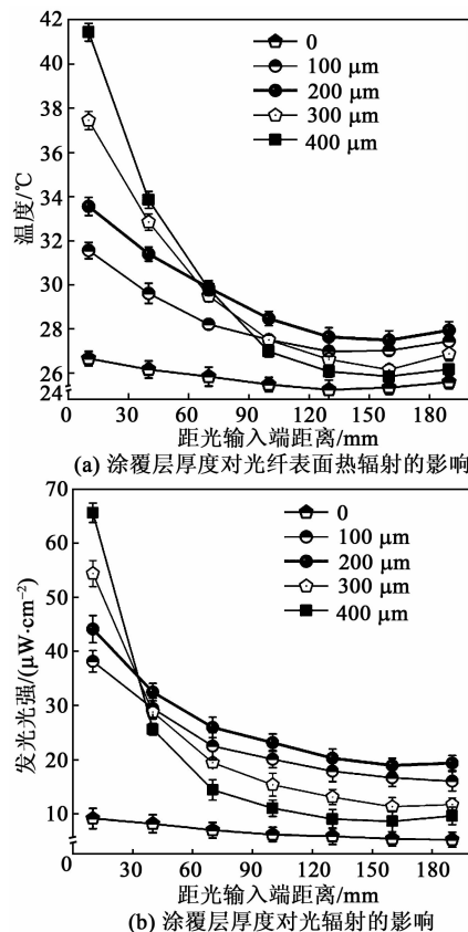
图5 w(\text{LaB}_6)=0.30\% 时,涂覆层厚度对光纤表面热辐射及光辐射性能的影响
