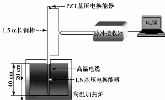
图 4 LN 基压电换能器高温性能测试装置
