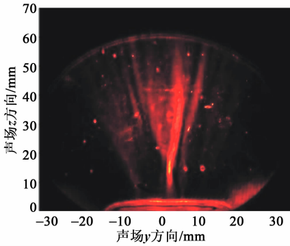
图 9 声场聚焦于(0,3 mm ,15 mm)的 Schlieren 像
