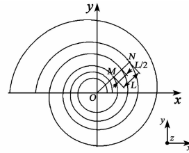
图6 螺旋电极线布置图
