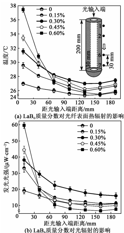
图4 涂覆层厚为 100\ \mu\text{m} 时, w(\text{LaB}_6) 对光纤表面热辐射及光辐射性能的影响
