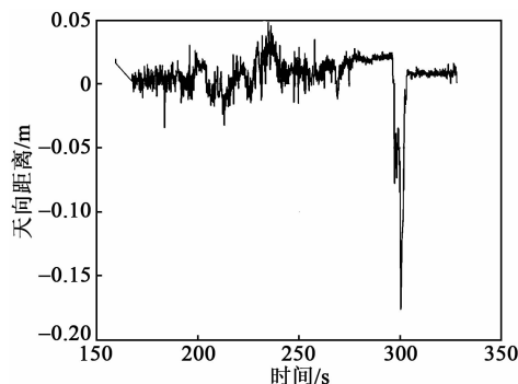
图 10 动态 RTK 相对定位天向距离曲线
