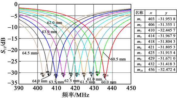
图 6 辐射体半径参数化扫描回波损耗变化
