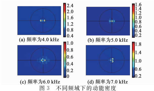
图 3 不同频域下的动能密度
