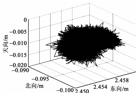
图 4 动 RTK 导航系统与基准站相对定位曲线
