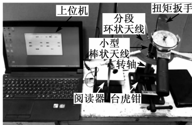
图 12 扭矩检测实验平台
