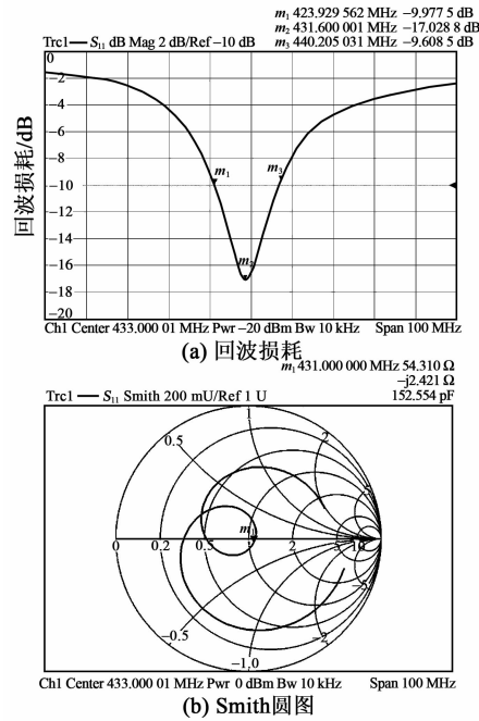
图10 天线测试结果
