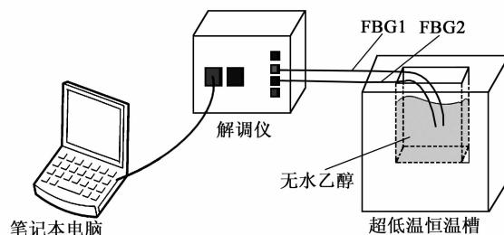
图3 实验装置图
