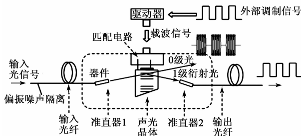
图1 光纤声光调制器原理图
