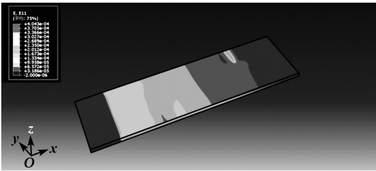
图 3 层间应变场
