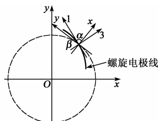
图 3 局部电极线结构坐标系
