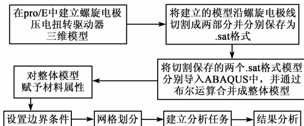
图 9 有限元分析流程图
