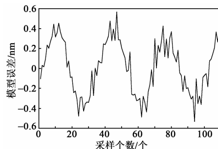
图5 f = 10 Hz时实际模型误差曲线
