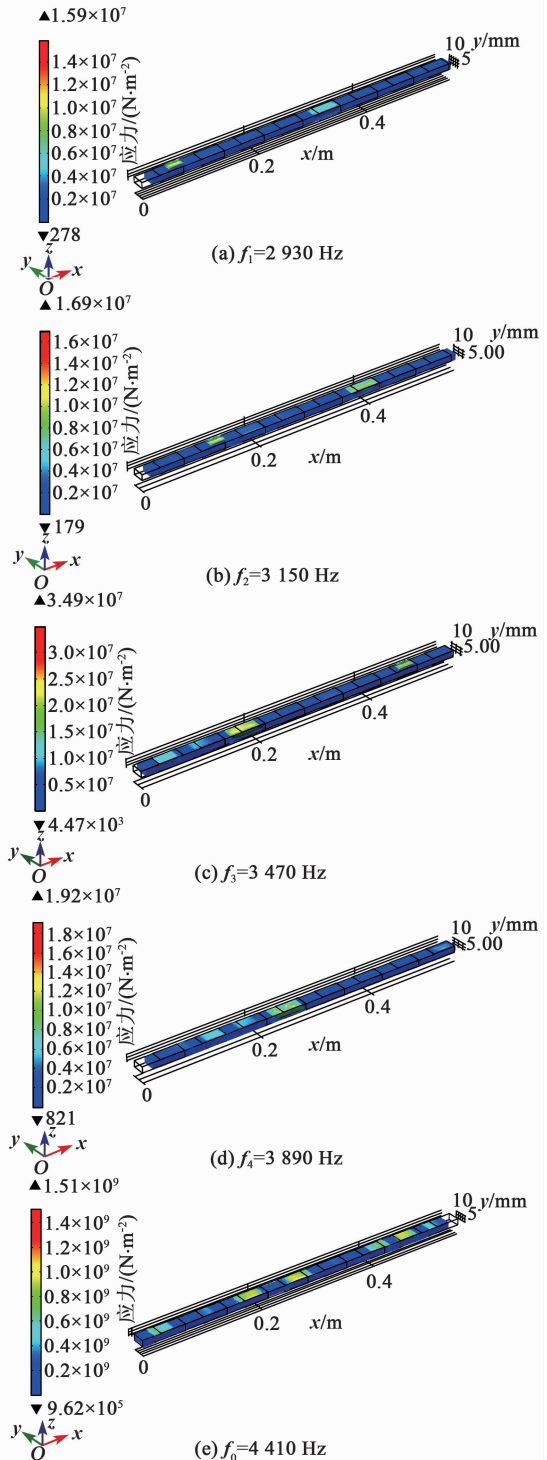
图7 不同频率下压电声子晶体杆的振型图
