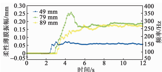
图8 柔性薄膜振幅曲线图
