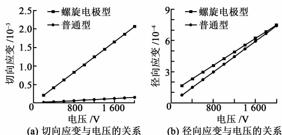
图 11 应变与电压的关系
