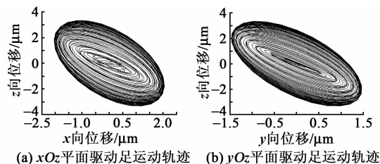
图8 驱动足在 xOz 、 yOz 平面内的椭圆运动轨迹
