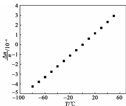
图2 石英材料 \Delta n/n 与 T 的关系图
