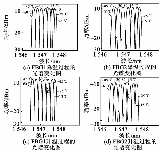
图4 FBG1、2随 T 变化的光谱变化图
