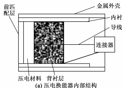
(a) 压电换能器内部结构
