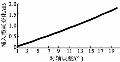
图 4 不同对轴误差对应的插入损耗变化
