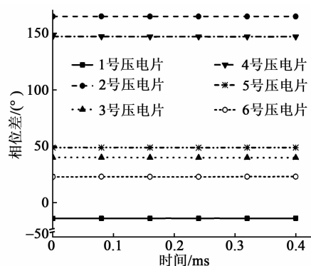
图10 单个压电片输出电压相位差图
