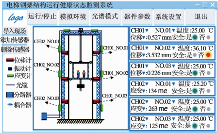
(b) 电梯钢接结构运行健康状态监测软件系统界面
