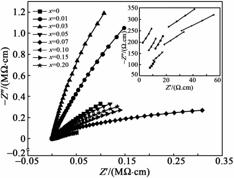
图 4 (Ca 0.97 Ba 0.03 )Cu 3 Ti 4-x Nb x O 12 陶瓷的室温阻抗谱
