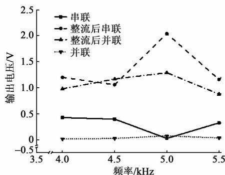
图12 直接串、并联及整流后串、并联压电片输出电压
