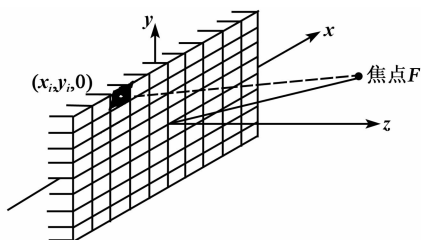
图1 二维相控阵
