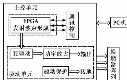
图2 超声相控阵控制系统框图
