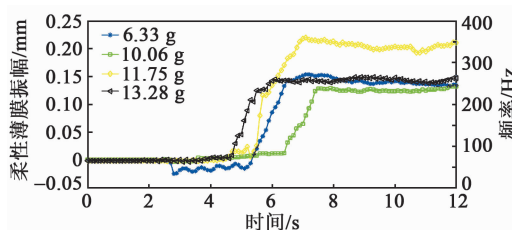
图6 柔性薄膜振幅曲线图
