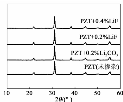
图1 x 、 y 不同时烧结样品的XRD图
