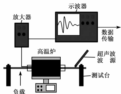
(b) YCOB基压电换能器高温接收性能测试装置
