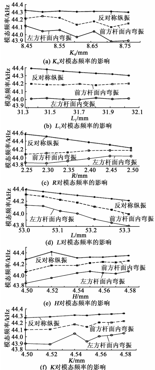
图 5 定子各特征尺寸对模态频率的影响
