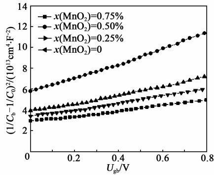
图 4 \text{SnO}_2\text{-ZnO-MnO}_2\text{-Ta}_2\text{O}_5 压敏陶瓷的 C\text{-}V 特性曲线
