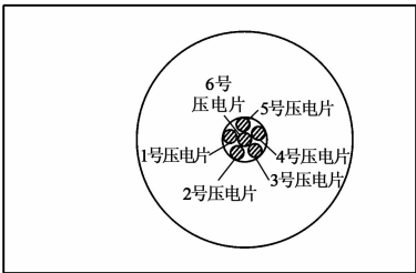
图 5 压电片摆放模型图
