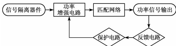
图4 驱动模块示意图
