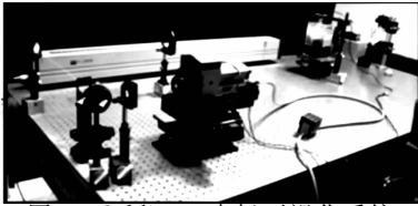
图 7 Schlieren 声场可视化系统
