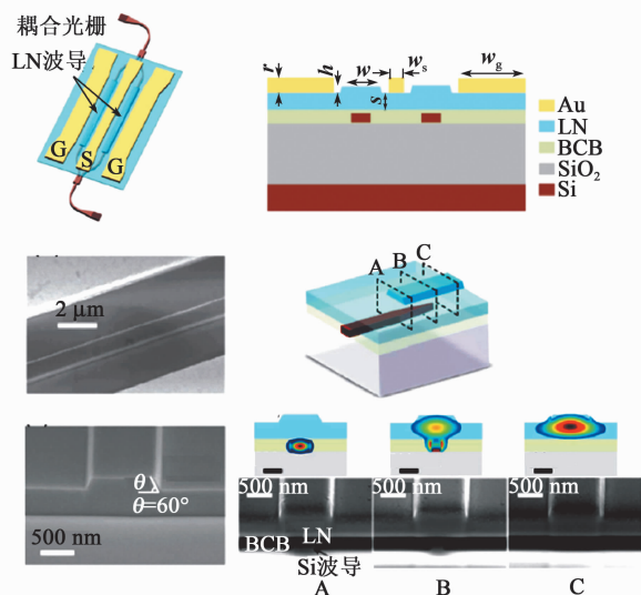
图 4 Si/LN 电光调制器
