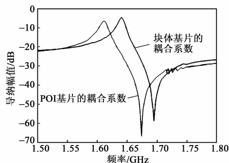
图9 POI 基片 SAW 谐振器和块体 LT 基片谐振器的耦合系数检测结果比较
