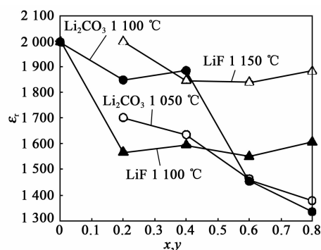
图8 烧结温度及 x 、 y 不同时样品的 \epsilon_r 图
