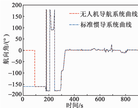
图 6 导航系统与标准惯导航向对比曲线
