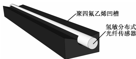
图 5 传感器封装示意图
