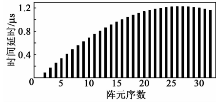
图4 各阵元上的时间延时图
