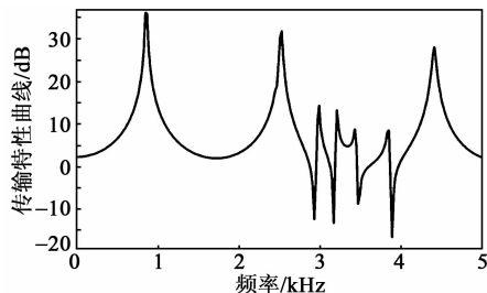
图6 COMSOL 计算传输特性
