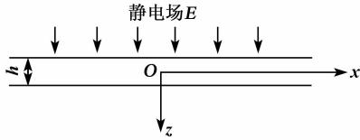
图 1 静电场中的压电薄膜
