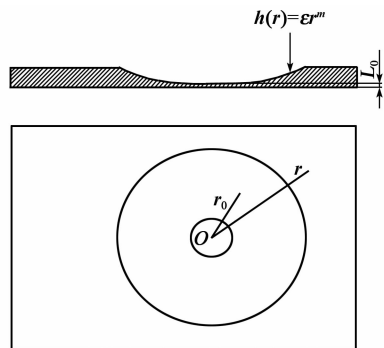
图 1 ABH 结构模型图
