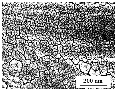
图 3 重复 50 次实验后钽膜结构扫描电镜图
