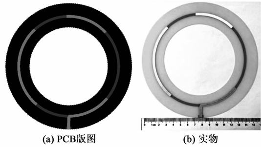
图9 实际制作的分段环状天线
