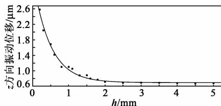
图 6 h 与缺陷处最大振动位移的关系
