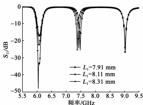
图 6 L_1 对滤波器通带的影响
