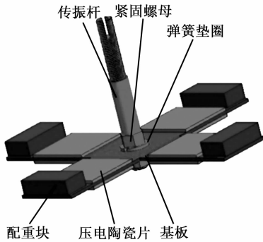
图1 压电惯性驱动器结构示意图
