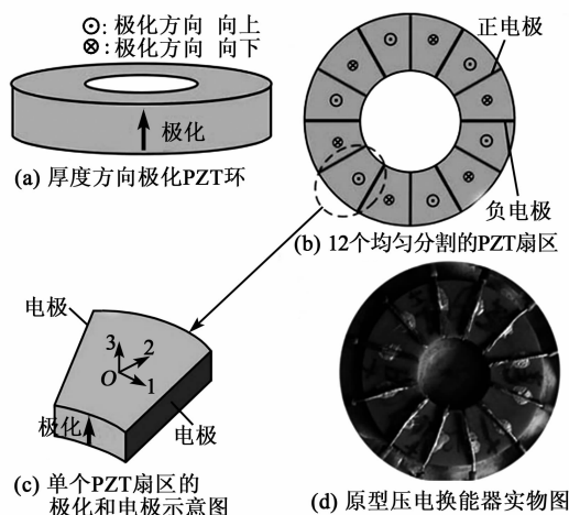
图2 压电圆环模型结构示意图
