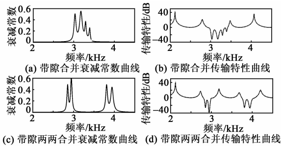
图5 配置Ⅲ型优化后的带隙结构及传输特性曲线
