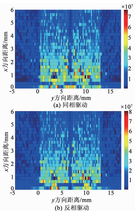
图6 中心频率 100 MHz 下两片换能器声辐射场分布图
