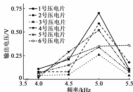
图11 单个压电片输出电压
