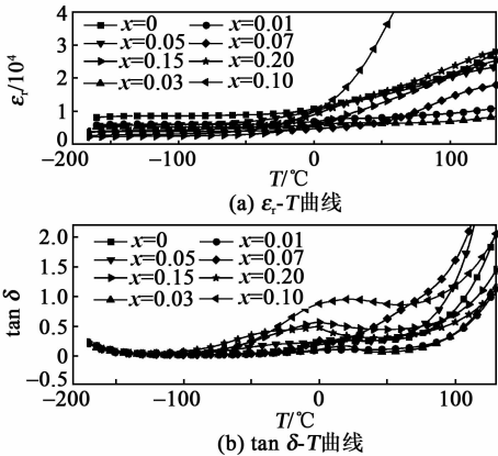
图 3 (Ca 0.97 Ba 0.03 )Cu 3 Ti 4-x Nb x O 12 陶瓷的介电温谱
