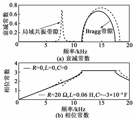
图3 压电声子晶体杆的带隙结构(配置 I)
