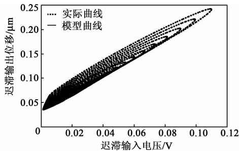
图 8 实际输出与模型输出曲线
