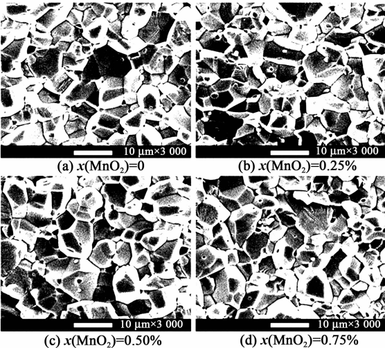
图 1 不同 x(\text{MnO}_2) 制备的 SnO 2 压敏陶瓷的 SEM 图像
