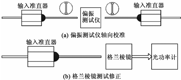
图 5 单偏振准直器调试工艺
