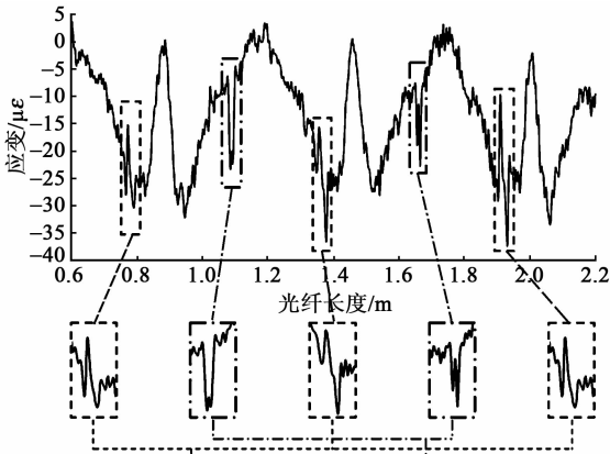
图 10 加载状态下试件应变
