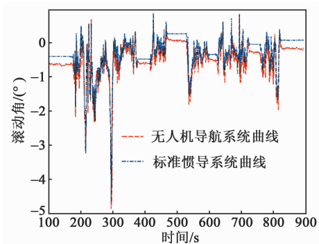
图 8 导航系统与标准惯导滚动对比曲线
