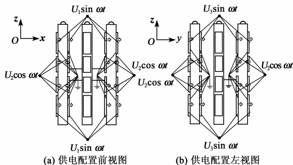
图 2 定子压电陶瓷极化供电配置
