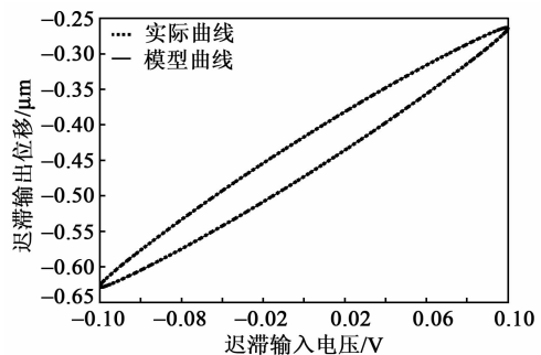
图2 f = 10 Hz时实际与模型输出曲线
