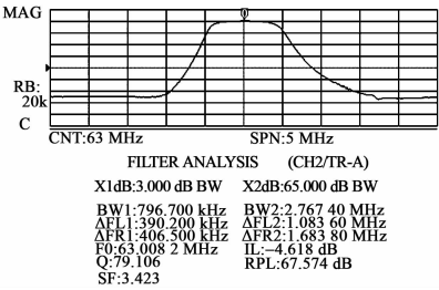
图 5 晶体滤波器实际指标
