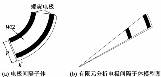
图 8 电极间隔
