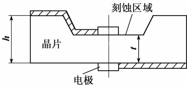
图 1 反台面晶体谐振器结构图
