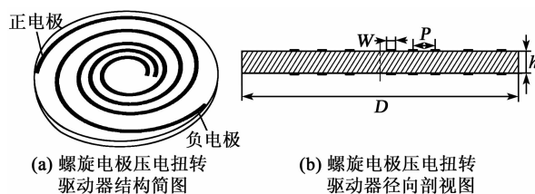
图 1 螺旋电极压电扭转驱动器结构图
