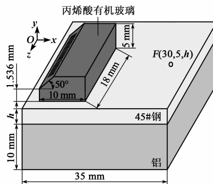
图 2 三维仿真模型示意图
