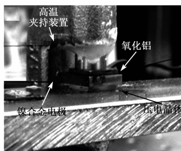
(a) YCOB基压电换能器与负载连接装置
