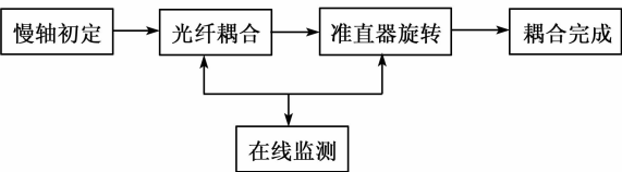
图 3 保偏光纤器件耦合方法
