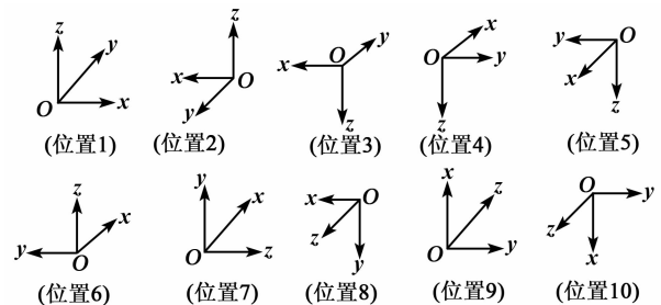
图 1 加速度计的 10 位置标定路径
