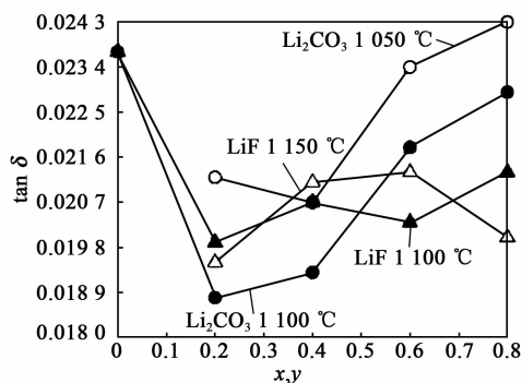
图9 烧结温度及 x 、 y 不同时样品的 \tan \delta 图
